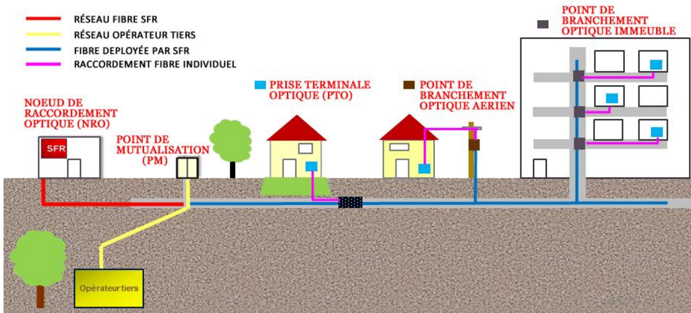
Schéma de principe du déploiement de la fibre
